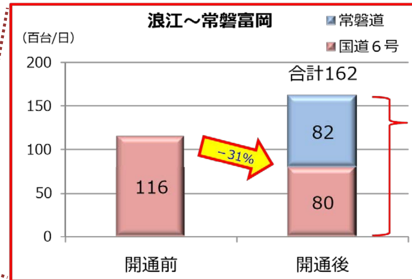
常磐自動車道全線開通後の交通量状況(開通後1ヶ月)
