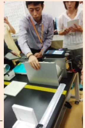
郡山市にあるWIZ国際情報工科大学校で。用途や厚みの異なる各種建築材料を試験した
