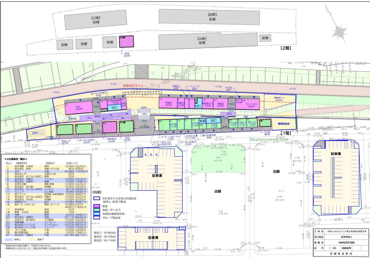
■商業施設・駐車場等整備計画図
