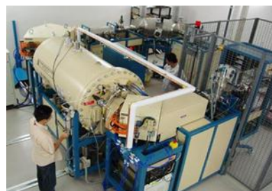
高精度質量分析装置。極微量の放射性核種の迅速分析を可能とする。
