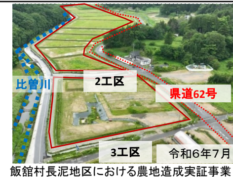
飯舘村長泥地区における農地造成実証事業
